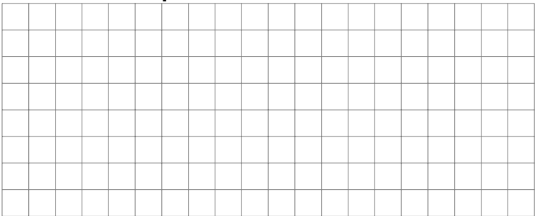
Propriété géométrique de la courbe parité de la fonction
